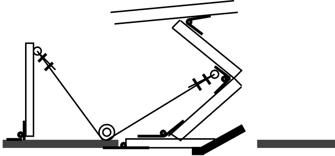
Spornbremse
